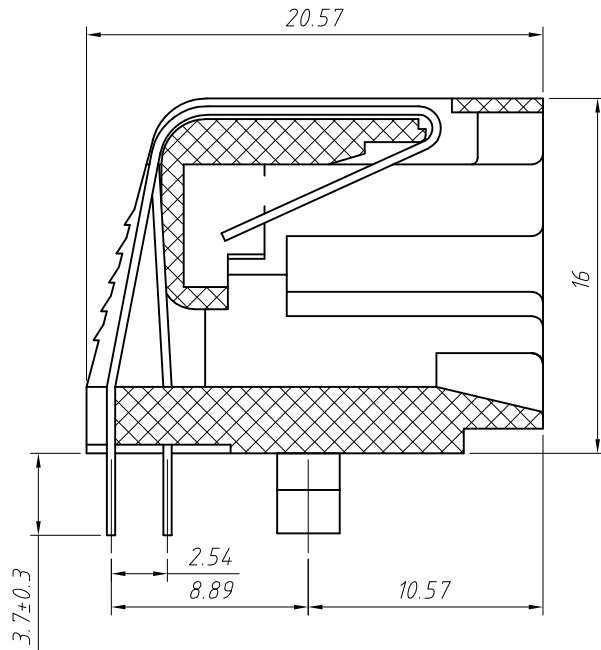
SECTION A-A
