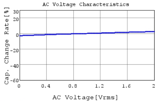
RCER71H104K0A2H03B C-AC Voltage capchange, I
