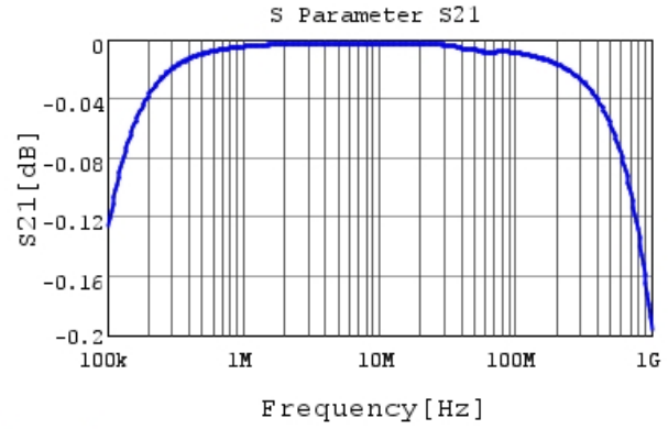
RCER71H104K0A2H03B S21 DC0V, 25degC
