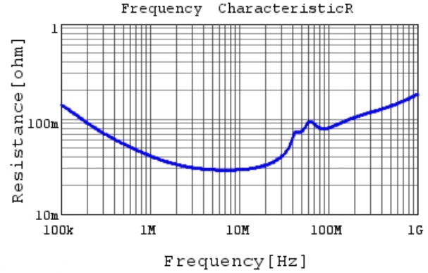
RCER71H104K0A2H03B R DC0V, 25degC
