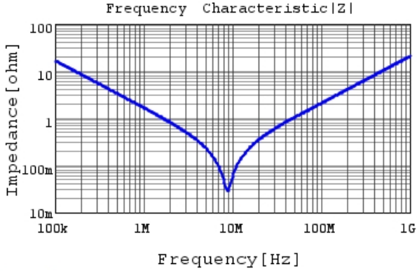
RCER71H104K0A2H03B |Z| DC0V, 25degC
