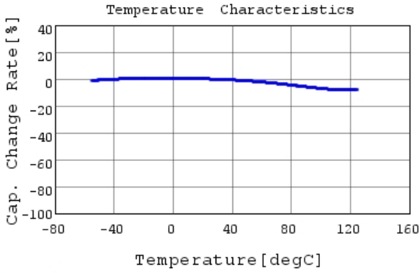
RCER71H104K0A2H03B C-Temp. capchange, DC0.0V
